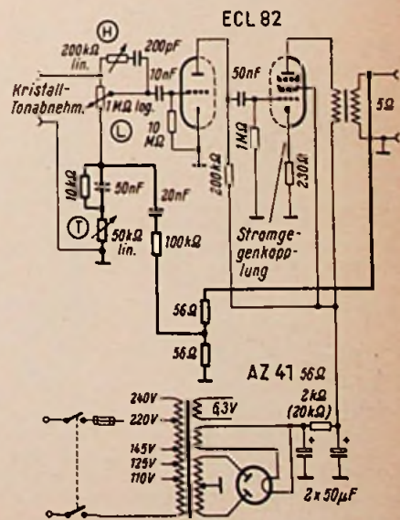
Bild 3. Schaltung eines Phono-Bar-Verstärkers
