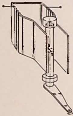
Bild 5. Bei dem neuen magnetodynamischen System von Philips induziert ein quermagnetisierter Ferroxid-Stab die Tonspannungen in den Spulen auf einem Weicheisenkern
