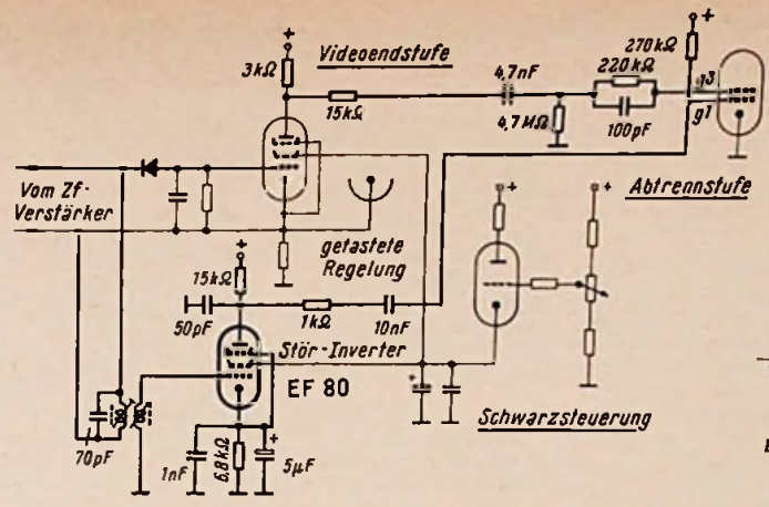
Bild 32. Schematisiertes Störpektrum an der Anode des Störinverters Rechts: Bild 33. Prinzipschaltung des Störinverters
