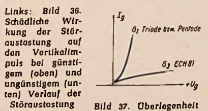
Bild 37. Überlegenheit der Gitterstromkennlinie am Gitter 3 der ECH 81 gegenüber der Gitterstromkennlinie einer Triode oder Pentode für die Abtrennung
