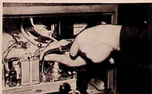
Bild 9. Unzugängliche Schrauben lassen sich mit diesem oolllsolierten Schraubenzieher mit biegsamem Schaft bequem lösen. (Friedrich Damm, Remscheid)
