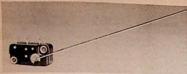
Bild 5. Dieser einpolige und sehr leicht ansprechende Drehumschalter mit Fühlhebel in Kleinformat für eine Wechselspannung bis 250 V kann bis zu 5 A belastet werden (Harting)
