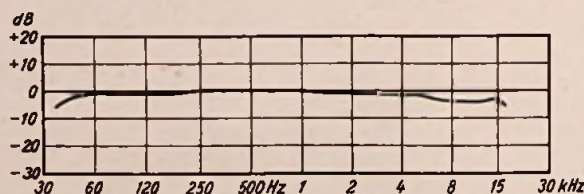
Bild 7. Frequenzgang des keramischen Tonabnehmersystems 3 TS (Telefunken). Die Kapsel wurde an einen Entzerrverstärker mit einem Eingangswiderstand von 840 kΩ über ein Meßkabel von 360 pF Kapazität angeschlossen
