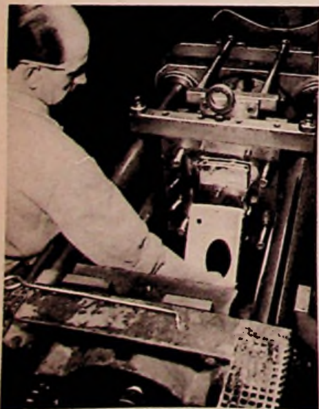
Bild 7. Eine der schweren Spritzgußmaschinen bei Grundig, die Kunststoff-Gehäuse samt eingesetzten Metallteilen in einem Arbeitsgang herstellen
