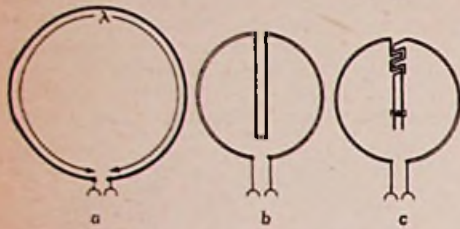
Bild 2. Wie die Fuba-Fernseh-Zimmerantenne Kiebitz entstanden ist
