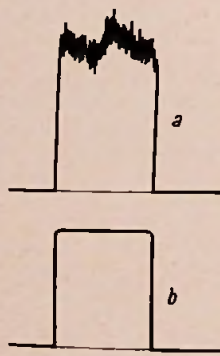
Bild 30. a = Störimpuls mit höherfrequenten Störspitzen, b = höherfrequente Störspitzen im Zf-Verstärker begrenzt
