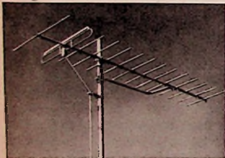
Bild 3. Einkanal-Antenne für Band III mit extrem hohem Gewinn und gutem Vor/Rück-Verhältnis (Kathrein-Gigant mit 14 Elementen)
