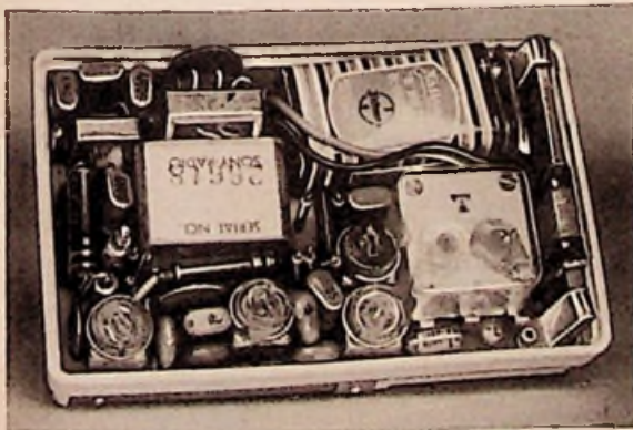
Bild 3. Innenansicht des Taschensupers
