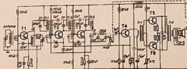
Bild 2. Schaltung des Taschensupers Sony
