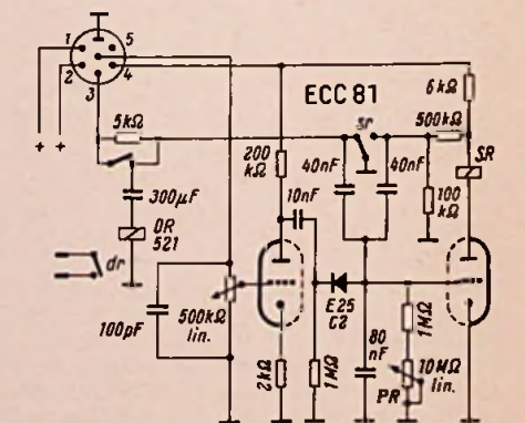
Bild 9. Schaltung des Acustomat D für automatische Dia-Projektion
