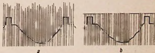
Bild 26. Zündstörungen auf dem Videosignal, a = unbegrenzt, b = begrenzt und abgeschnitten
