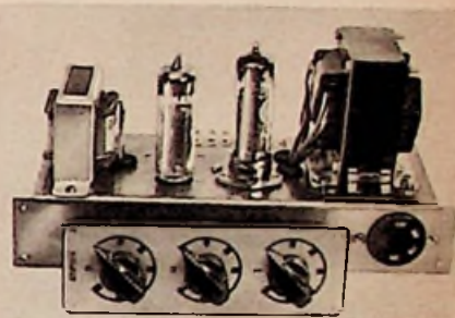
Bild 2. Phono-Bar-Verstärker in Chassis-Ausführung (Klein & Hummel)
